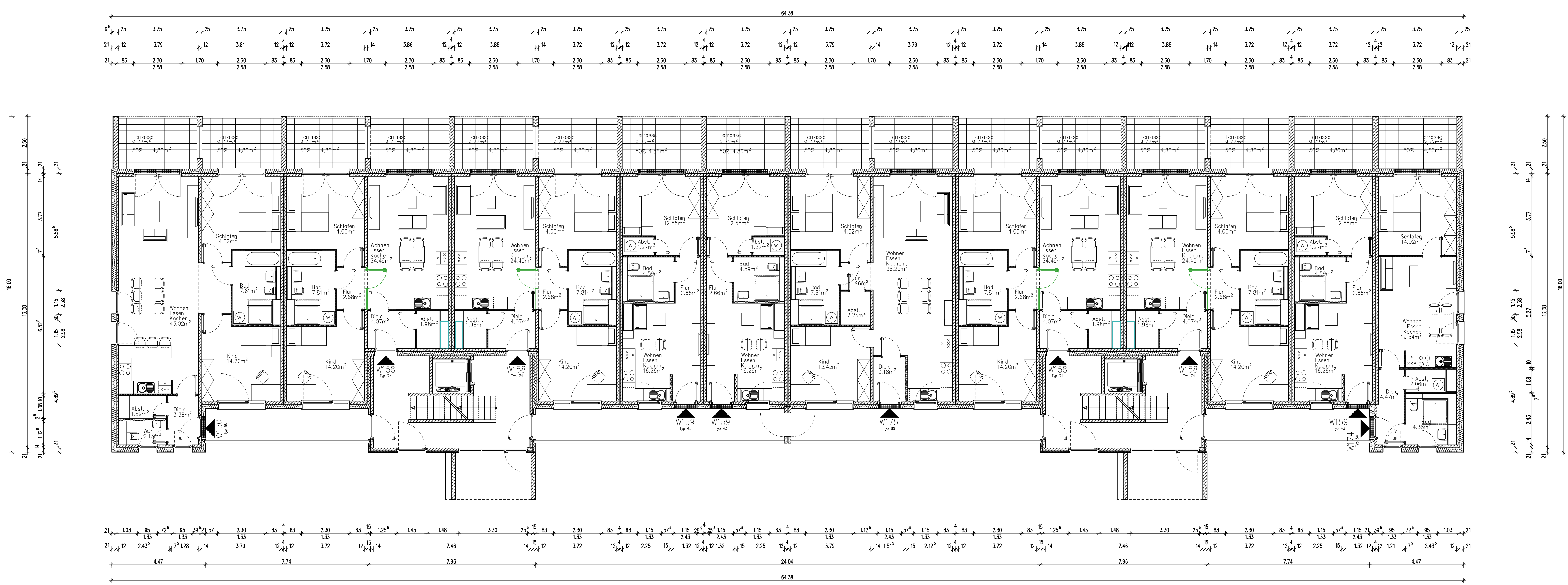
ERDGESCHOSS 1:100
